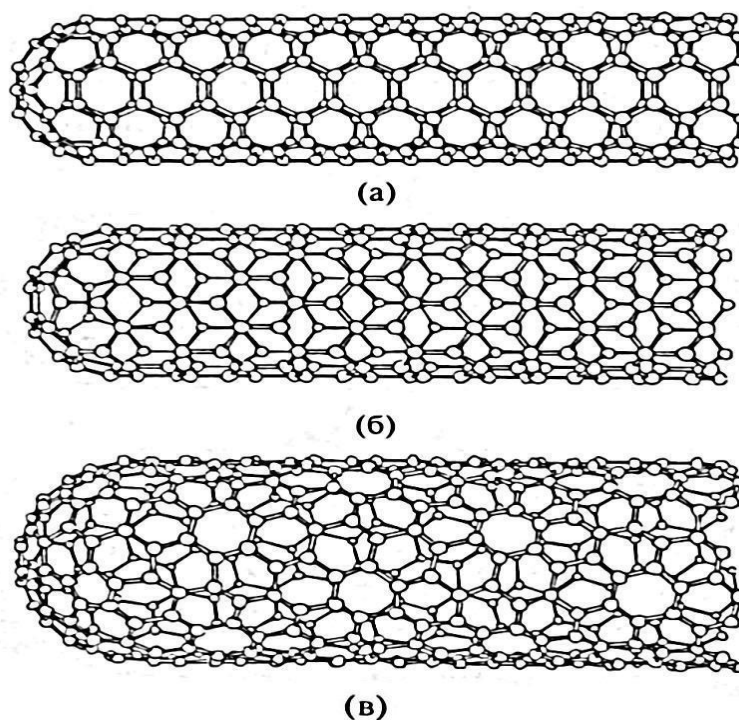
Сурет 4.2 - Көміртегі нанотүтік: а – "кресло" типті; б – "зигзаг" типті; в – хиральді КНТ
